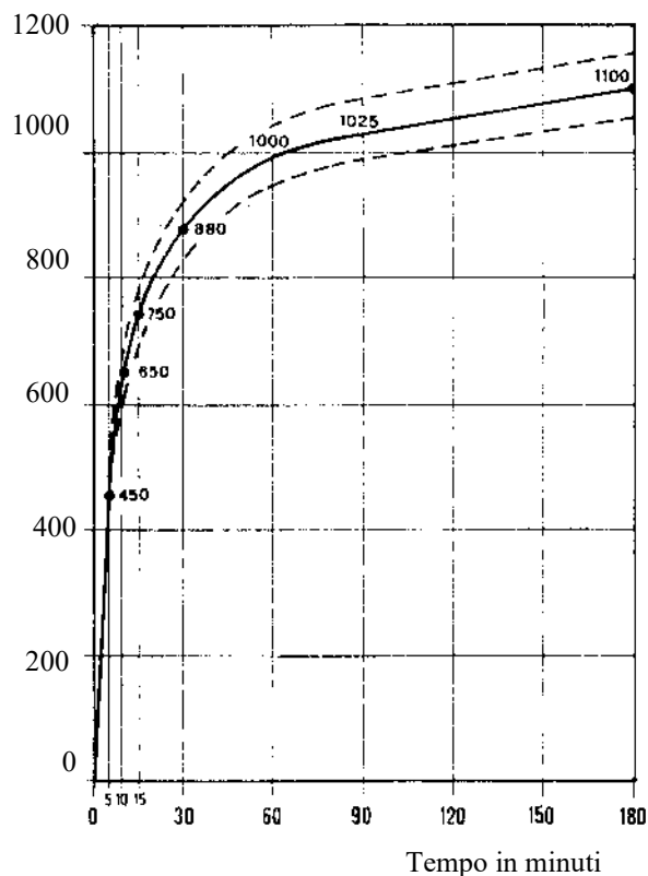
Fig. 2 – Curva temperatura - tempo.
