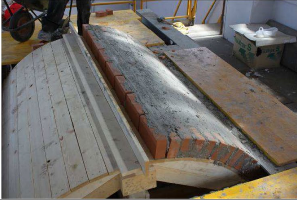
14/5/2015 – figura 30 Completamento della prima metà della volta muraria
