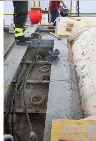
15/5/2015 – figura 33 Posizionamento delle termocoppie interne in corrispondenza della sezione di imposta alle reni
