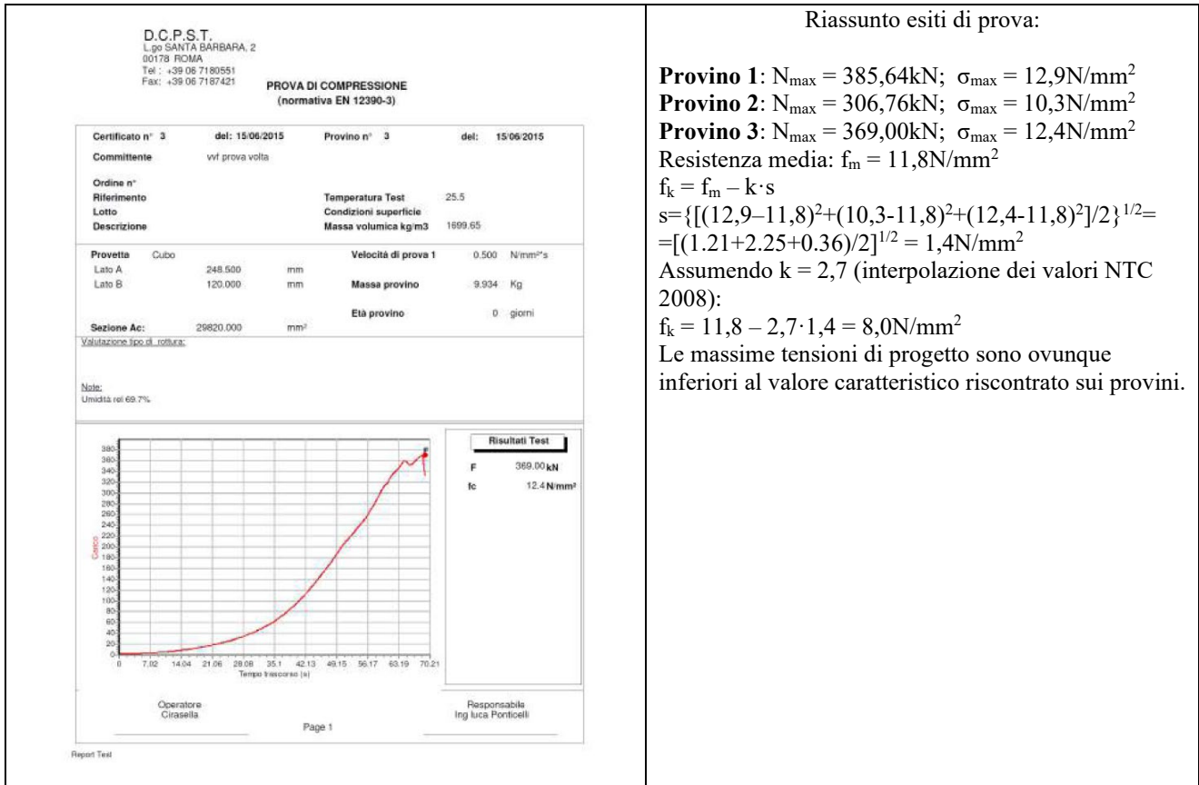
Figura 60 – Esiti delle prove di compressione sui provini di muratura
