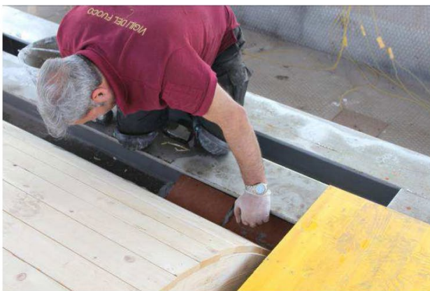
13/5/2015 – figura 28 Inizio della realizzazione della prima metà volta muraria a partire dalla sezione di imposta alle reni
