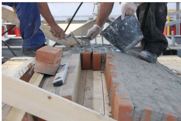
18/5/2015 – figura 36 Chiusura della chiave della volta
