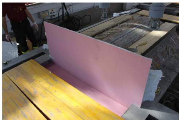
16/6/2015 – figura 55 Tamponatura frontale della volta con lana di roccia e cartongesso
