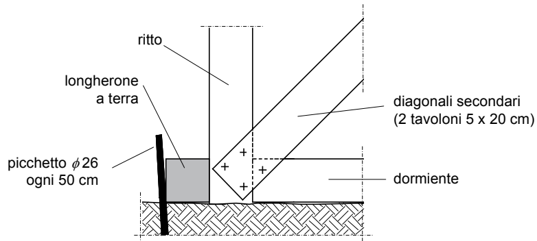
SEZIONE VERTICALE
