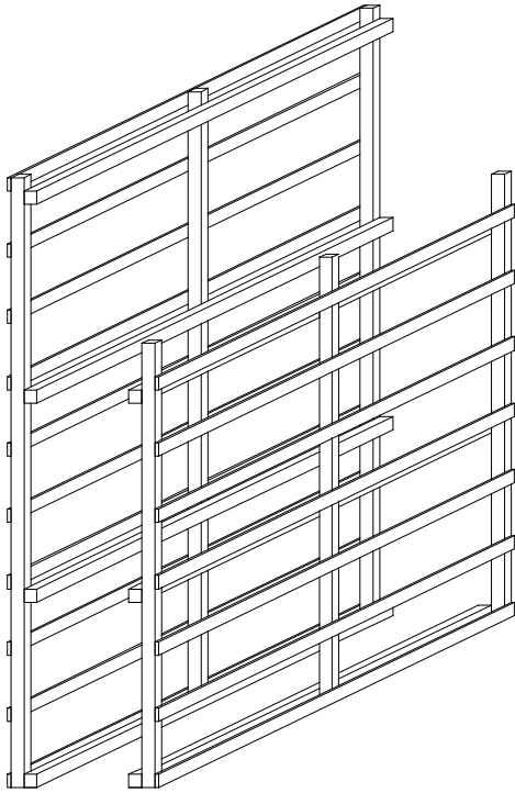
Fase 1 – Realizzazione dei graticci di ripartizione
