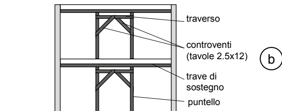
Sezione trasversale
