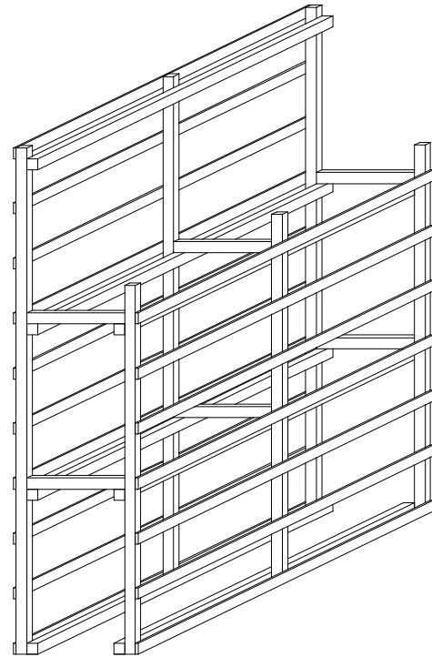
Fase 2 – Collegamento trasversale dei graticci
