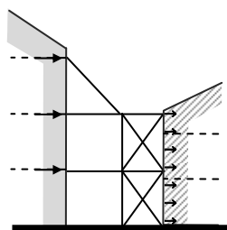
Sezione verticale
