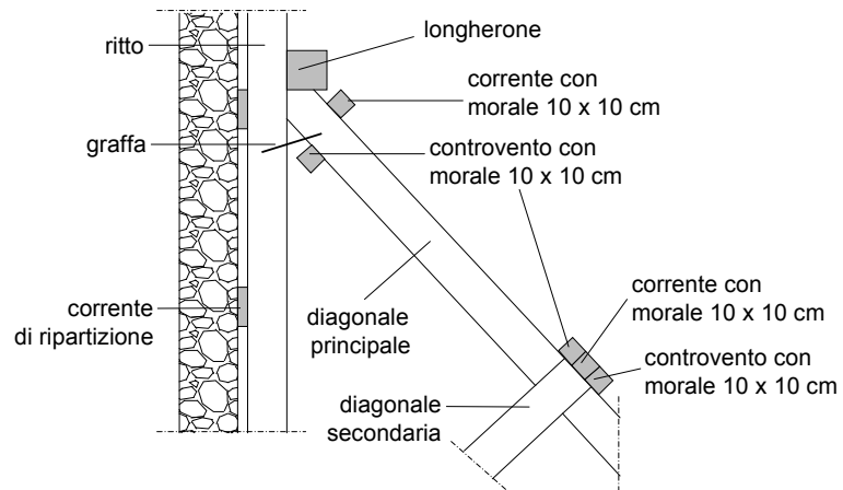
SEZIONE VERTICALE
