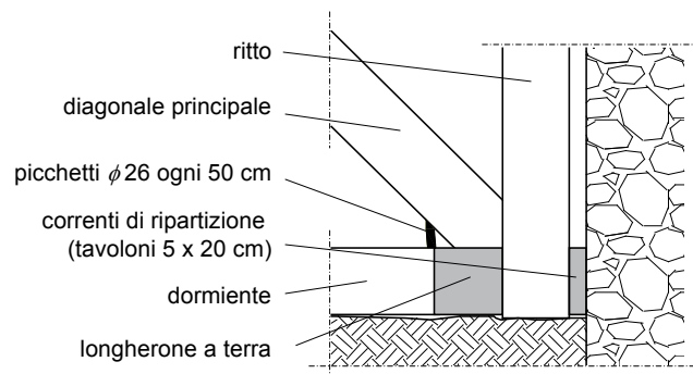
SEZIONE VERTICALE
