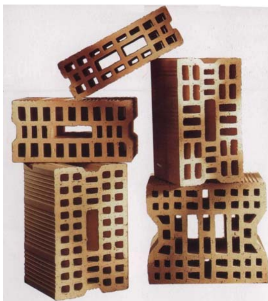
Figura 2.12 Laterizi forati
