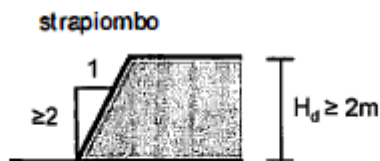
Figura 1 - Caratteristiche geometriche di un dislivello a strapiombo
