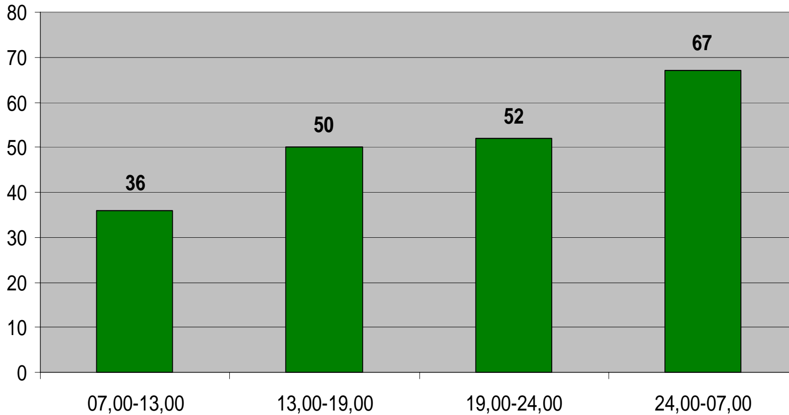
Suddivisione oraria degli incendi di grande rilevanza negli alberghi e simili in Italia dal 1990 al 2008
