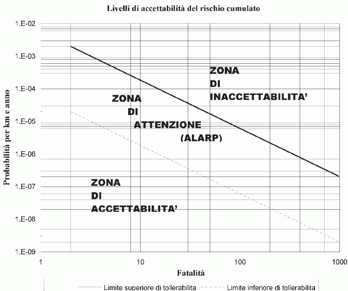
Tavola 4.3.1: Obiettivi di sicurezza: livelli di accettabilità del Rischio Cumulato nelle gallerie ferroviarie. Il dato della probabilità di superamento 1-F(x) è normalizzato rispetto ai chilometri di percorrenza annua sulla rete.
