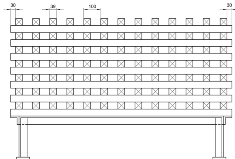
figura 1.2 Esempio di focolare di classe A (focolare 13 A) - Vista laterale (variabile secondo le dimensioni del focolare) Dimensioni in millimetri
