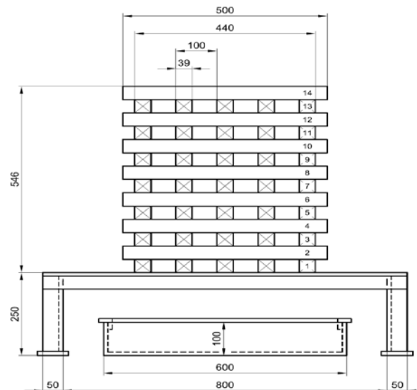
Esempio di focolare di classe A (focolare 13 A) - Vista frontale (Identica per tutti i focolari) Dimensioni in millimetri
